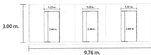
ตัวเวทีตั้งบนแผงฉากหน้าเวที
